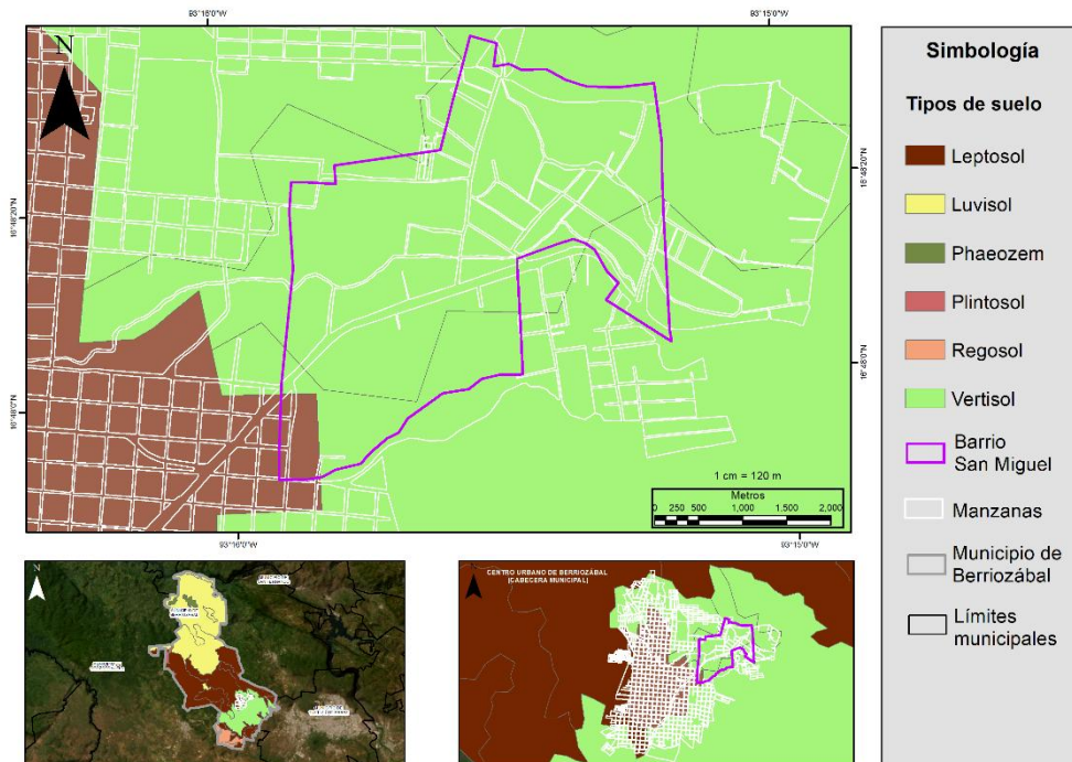
Mapa edafológico del barrio San Miguel, municipio de Berriozábal, Chiapas.
